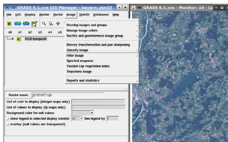
Abb.1: Tcl/TK basierter GIS-Managerr
